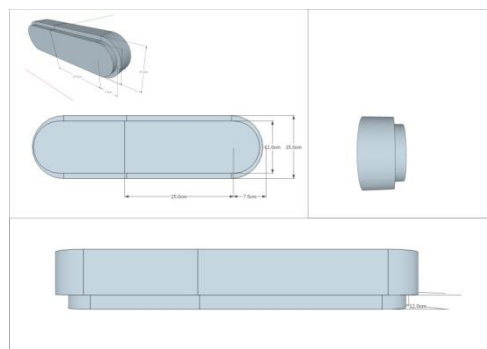
Gambar 2 Desain Rekomendasi Tutup V- belt
