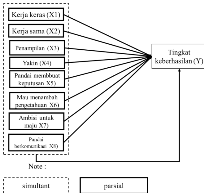
Gambar 1 Kerangka berpikir
