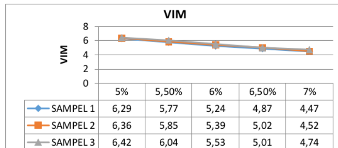
Gambar 2. Nilai VIM.
