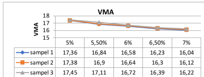
Gambar 1. Nilai VMA.
