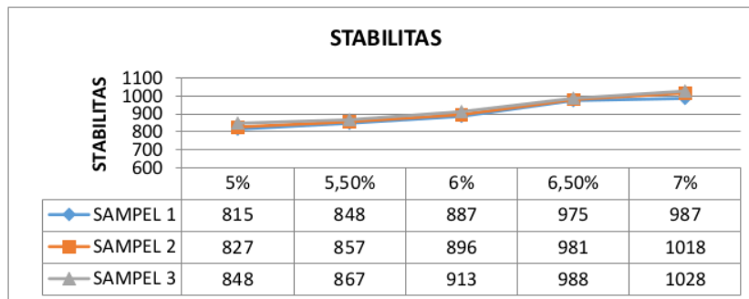
Gambar 4. Nilai Stabilitas.
