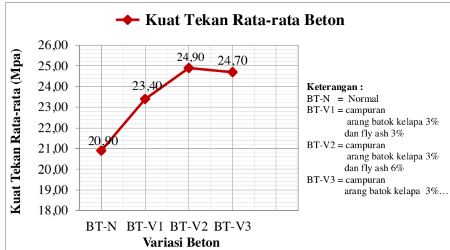
Gambar 4. Grafik Uji Kuat Tekan Rata-rata
