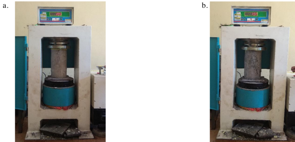
Gambar 8. (a) Proses Tes Kuat Tekan (b) Benda Uji Hancur
