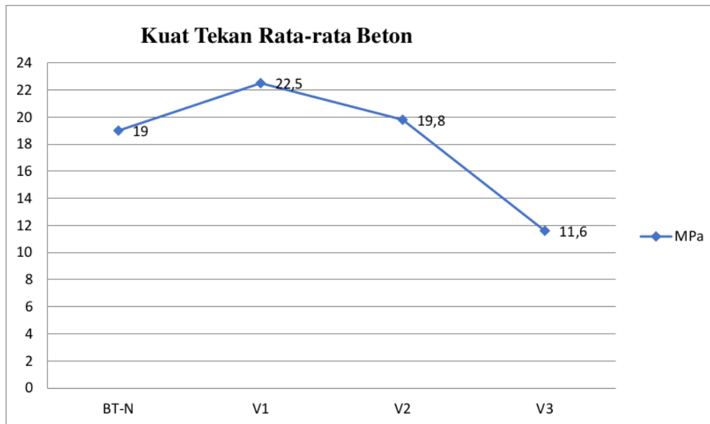
Gambar 7. Grafik Hasil Pengujian Kuat Tekan Rata-Rata Beton
