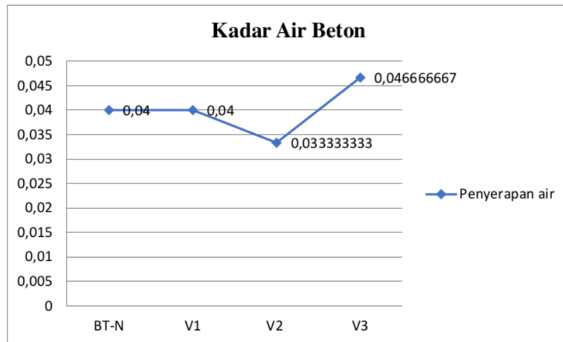
Gambar 9. Grafik Hasil Pengujian Kadar Air
