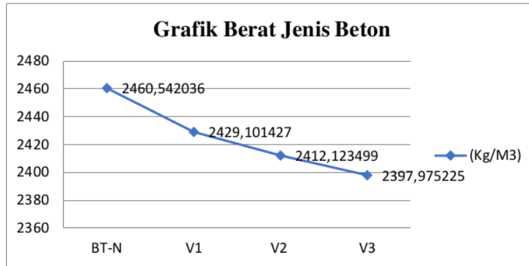
Gambar 10. Grafik Hasil Pengujian Berat Jenis Beton
