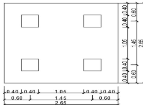
Gambar 5. Tiang Pancang Square Pile 40 x 40 Tipe P-1.
