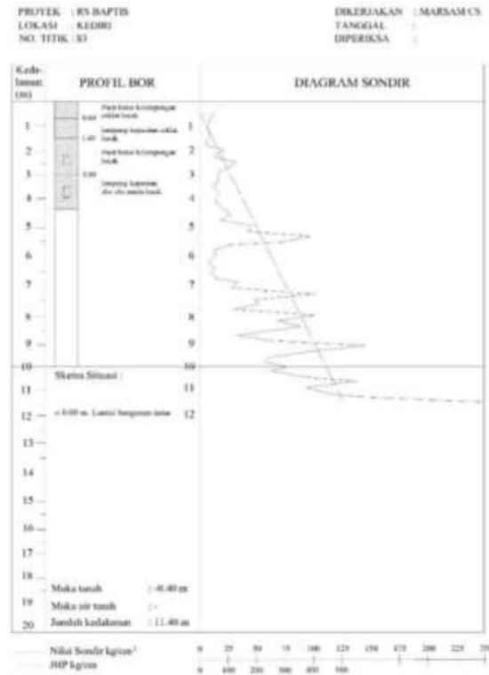
Gambar 4. Data Sondir RS Baptis Kediri.
