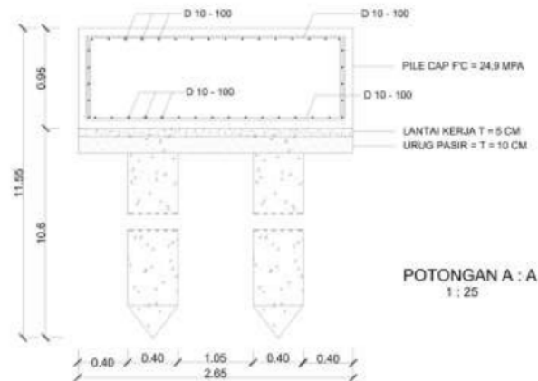
Gambar 6. Pengaplikasian penggunaan pile cap dengan tulangan D10-100
