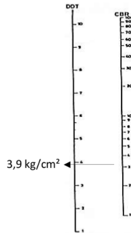
Gambar 1. Grafik Korelasi Penentuan DDT.
