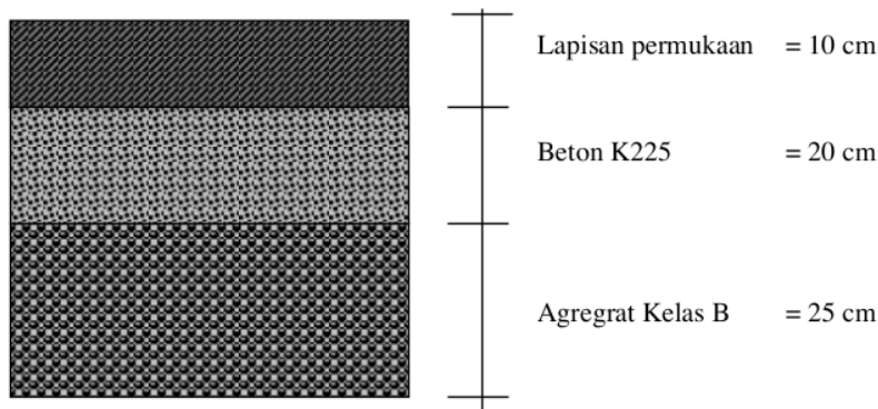
Gambar 2. Ketebalan perkerasan rencana
