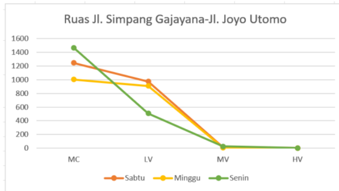
Gambar 4. Grafik Jumlah Lalu-Lintas Harian di Jl. Simpang Gajayana – Joyo Utomo.
