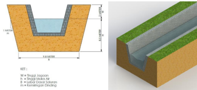
Gambar 4. Desain Drainase Saluran Berbentuk Trapesium
