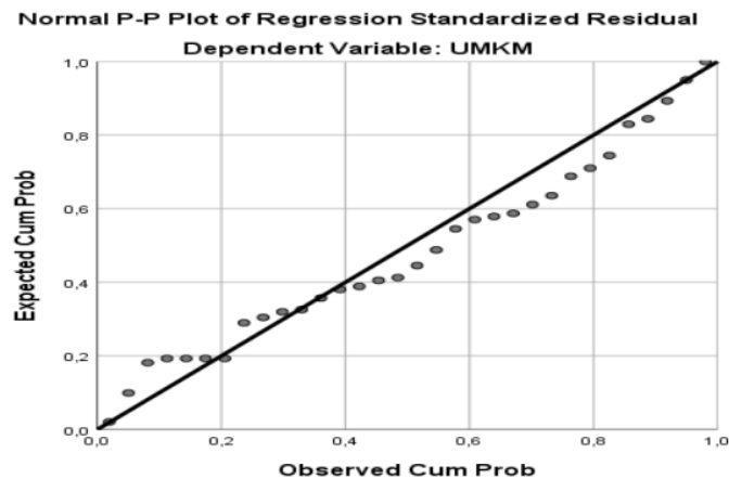
Gambar 1. Grafik P-Plot Uji Normalitas
