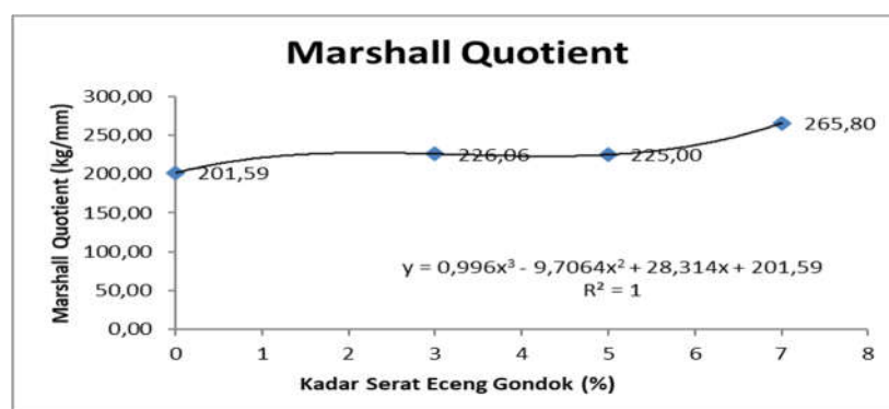
Gambar 9. Grafik Hubungan Marshall Quotient dengan Kadar Serat Eceng Gondok
