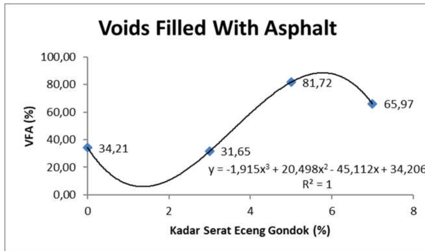
Gambar 4. Grafik Hubungan Voids Filled With Asphalt dengan Kadar Serat Eceng Gondok Sumber : Hasil Perhitungan, 2018
