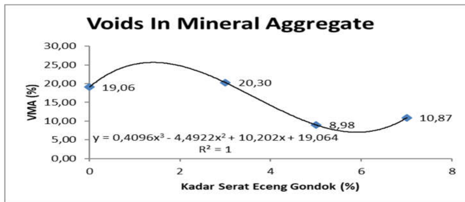
Gambar 6. Grafik Hubungan Voids In Mineral Agregate dengan Kadar Serat Eceng Gondok Sumber : Hasil Perhitungan, 2018
